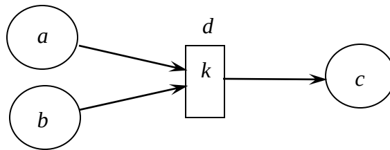
Рис.1(в). К-сеть удаляющего перехода d: a, b > c: k : тип 6,7,8;
