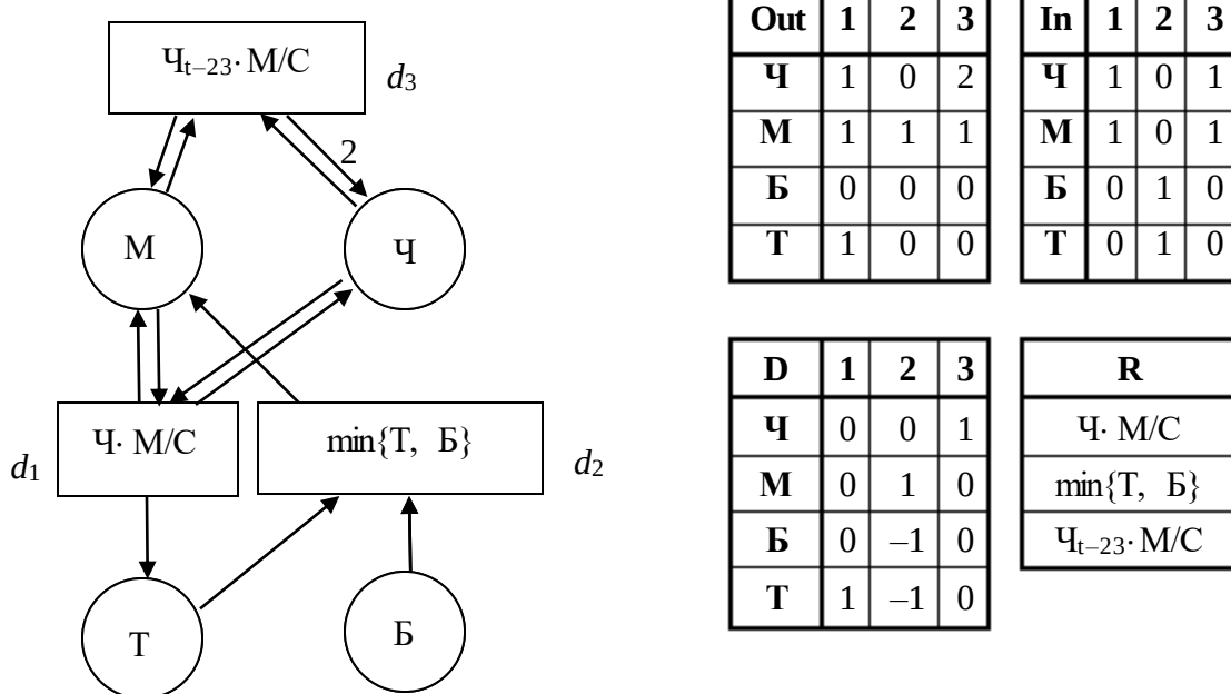
Рис. 6 (б). К-сеть и матричное представление демографического процесса.
