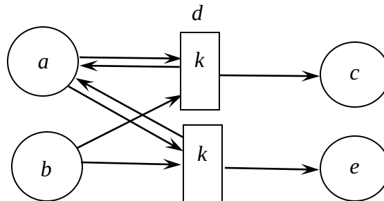
Рис.1(г). К-сеть остаточного перехода a: b > e: k : тип 9,10,11 в комбинации с простым переходом a: b > c: k : тип 0, 1, 2. Число состояний a сохраняется, все автоматы из b переходят в c и e .
