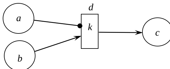
Рис.1(д). К-сеть перехода с ингибитором a: b > c: k : тип 0,1,2; Число состояний a сохраняется, b – убывает, c – увеличивается. Ингибитор изображён стрелкой с кружком на конце.
