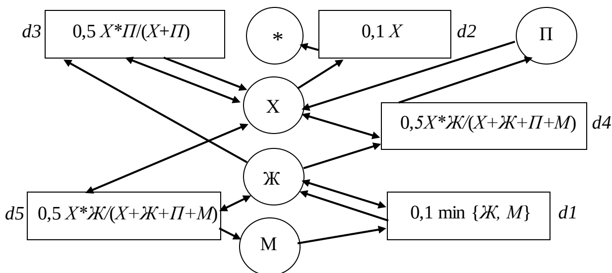
Рис.4. К-сеть хищник-жертва.
