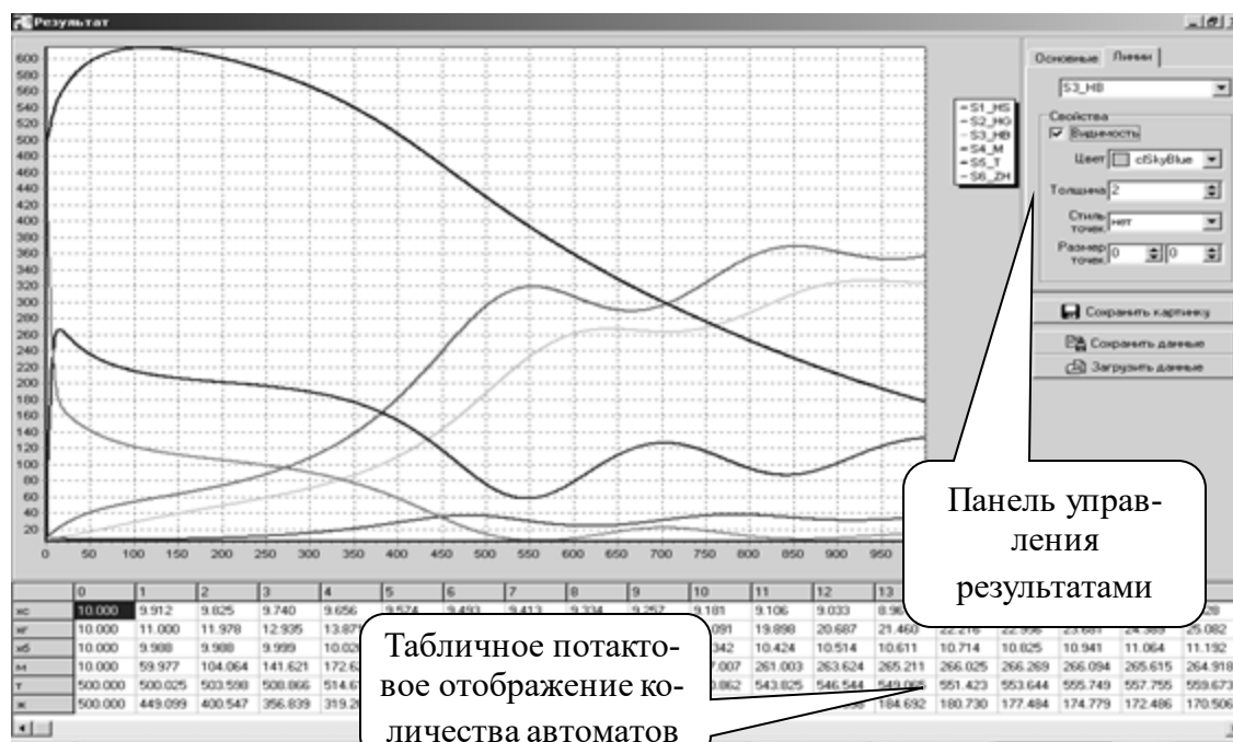
Рис. 9 (а, б). Главная форма и представление результатов моделирования
