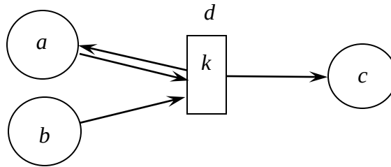
Рис.1(а). К-сеть простого перехода a: b > c: k : тип 0,1,2; Число состояний a сохраняется, b – убывает, c – увеличивается.
