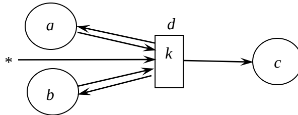
Рис.1(б). К-сеть сохраняющего перехода a, b: > c: k : тип 3,4,5; Число состояний a и b сохраняются, c – увеличивается. Внешнее состояние «*» не записывается в переход.
