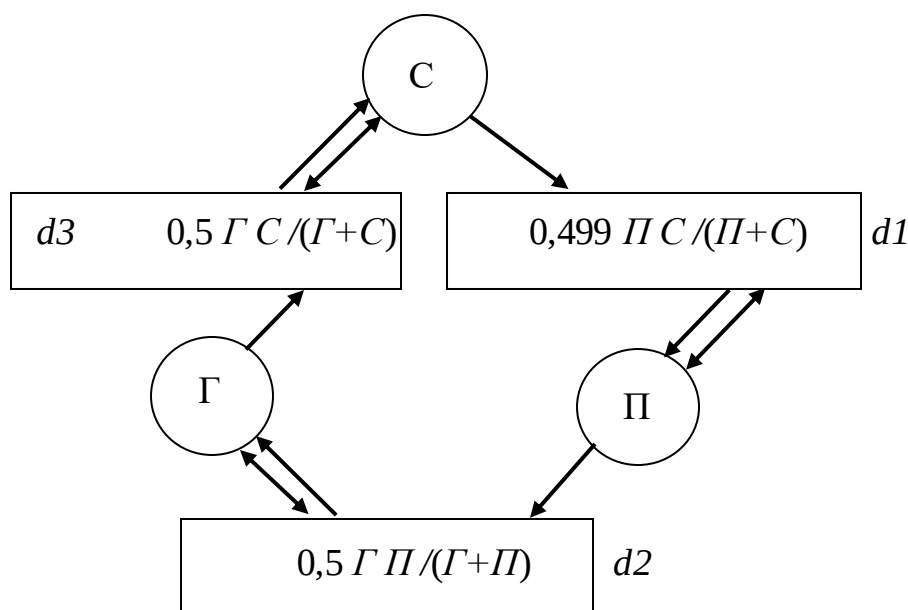
Рис. 8. К-сеть циклической пищевой цепочки в смеси.
