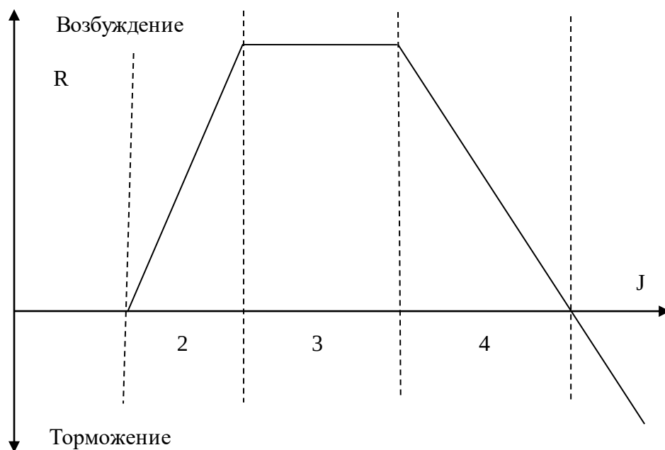
Рис. 3. Кривая Введенского.
